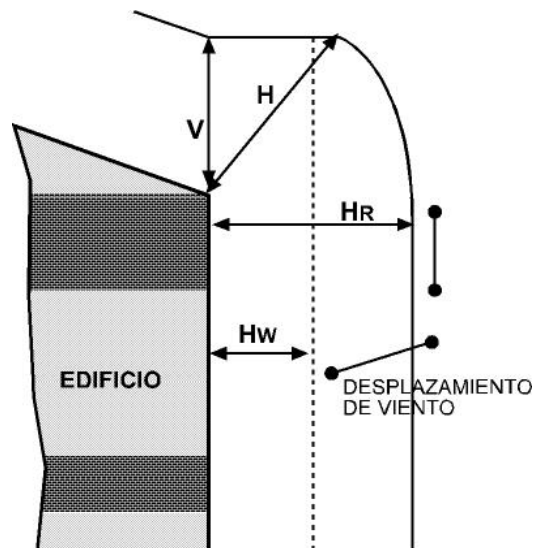
Figura No. 2 9 Distancias de Seguridad a Edificaciones
