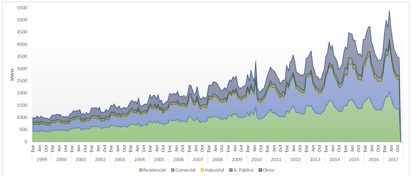
Figura 1. Demanda de energía eléctrica en Galápagos (enero 1999 – diciembre 2017) Fuente: ELECGALAPAGOS.
